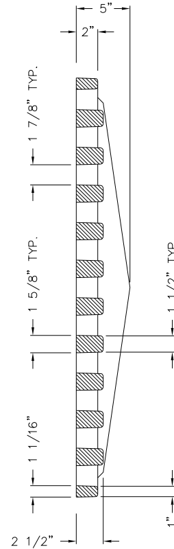
SECTION A-A
